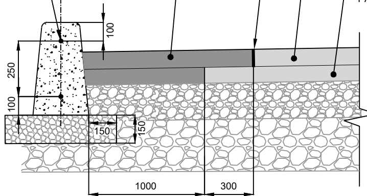
COUPE : BORDURE
