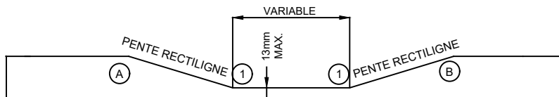
ÉLEVATION
